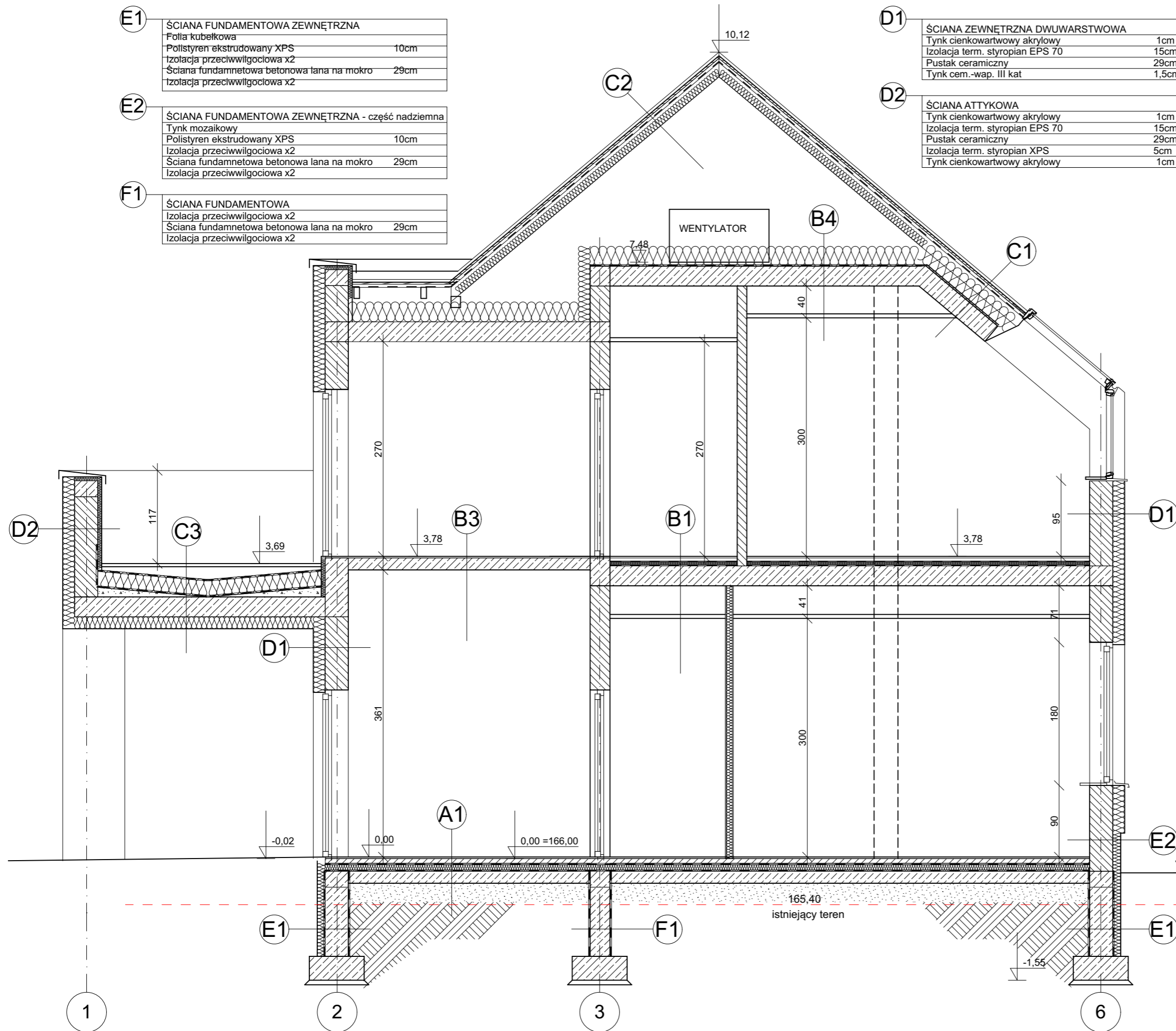
RZEKRÓJ B-B
